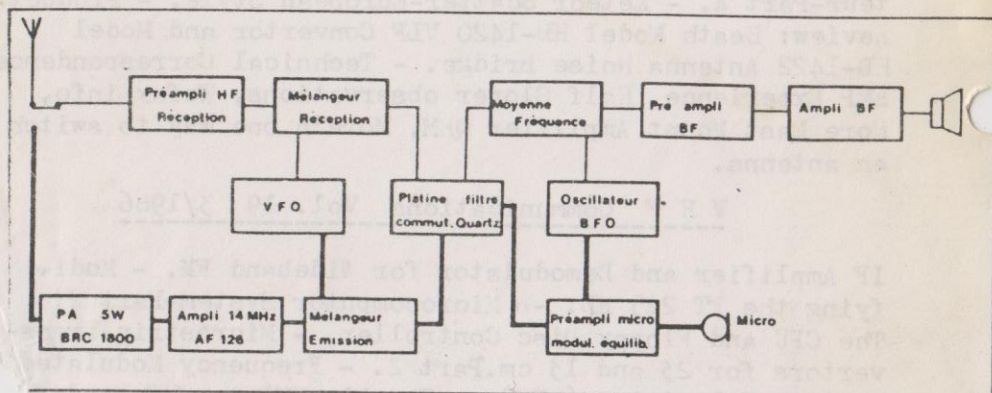
SYNOPTIQUE DU TRANSCIVER — ORGANISATION DES PLATINES
