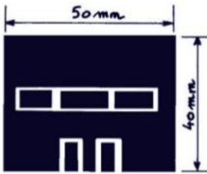
circuit imprimé filtre passe-bas
