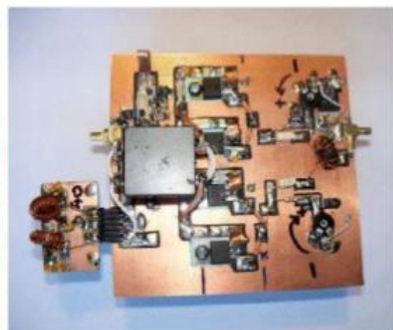
Détail de la disposition du filtre passe-bas enfichable en sortie du PA
