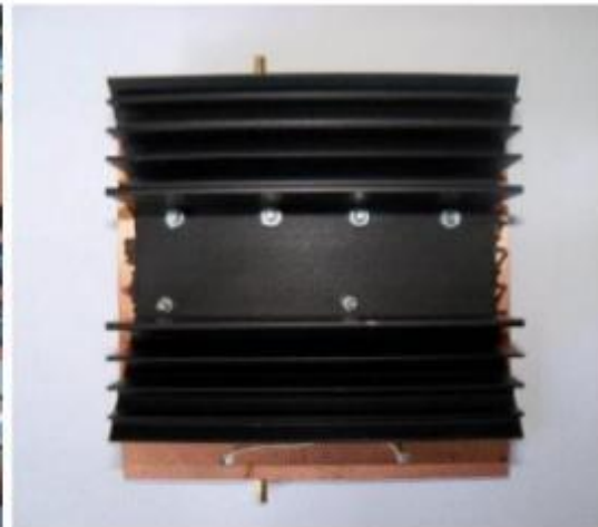
Il existe un radiateur de 10 x 10 cm et 3,8 cm d'épaisseur et de 5mm d'épaisseur disponible chez GOTRONIC sur le web
