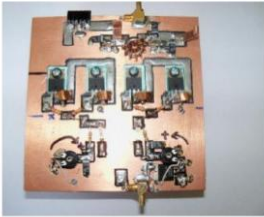
Les 4 x IRF510 sont isolés du radiateur par une lamelle en mica ou téflon isolant et canon de vis Ø 3mm en téflon.
