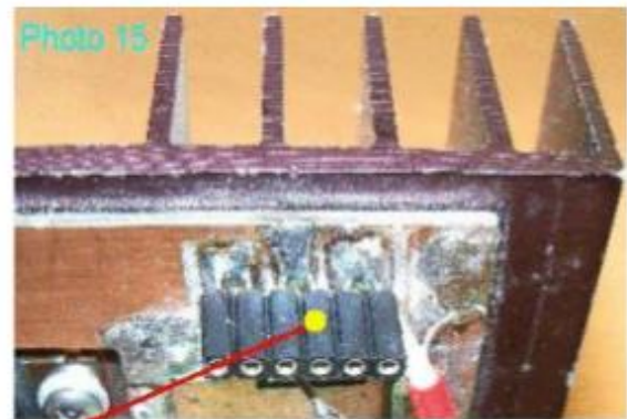
Connecteur H100 sur le P.A. Femelle
